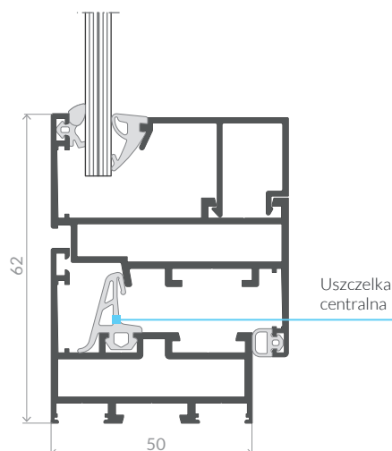
Przekrój przez okno otwierane
