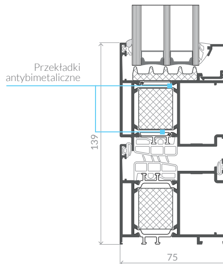
Przekrój przez drzwi otwierane do wewnątrz
