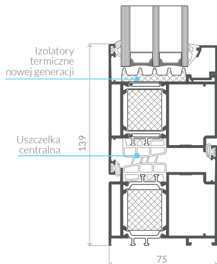
Przekrój przez drzwi otwierane na zewnątrz
